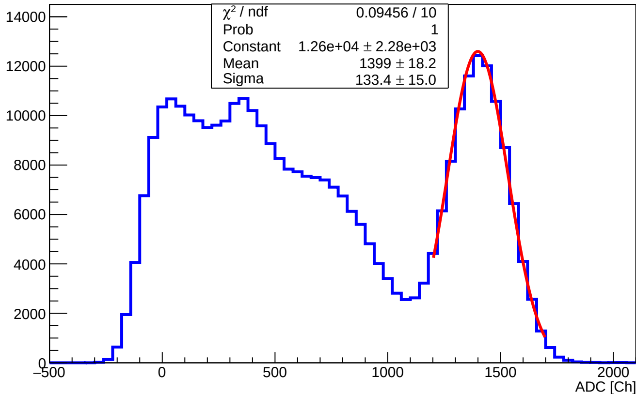
Spettro del ^{137}\text{Cs} con BGO, soglia a 15 mV e fit sul picco fotoelettrico
